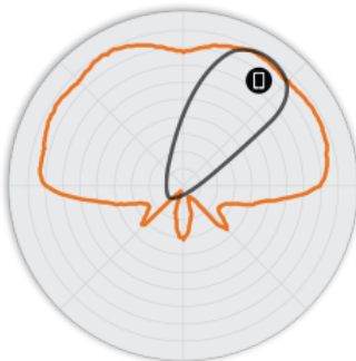
Figure 5. Diagrammes d'antennes Élévation 5 GHz
