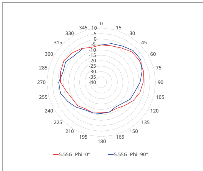
5.5 GHz (ANT1, 2, 3, 4)
