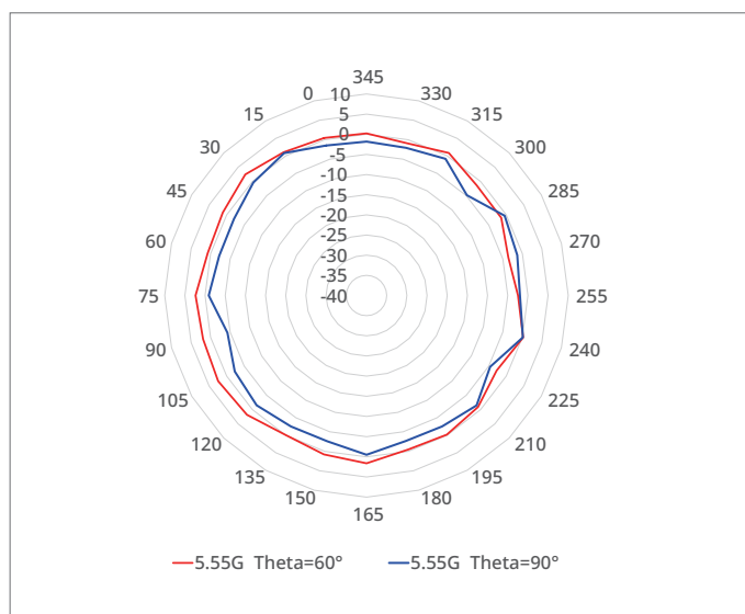
5.5 GHz (ANT1, 2, 3, 4)
