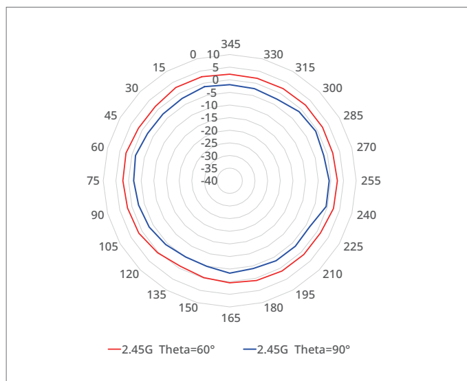
2.4 GHz (ANT1, 2, 3, 4)
