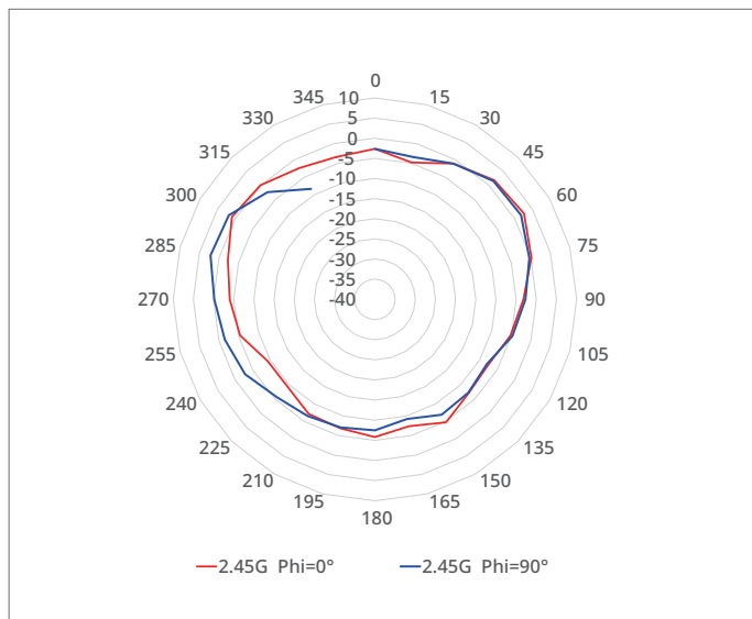
2.4 GHz (ANT1, 2, 3, 4)
