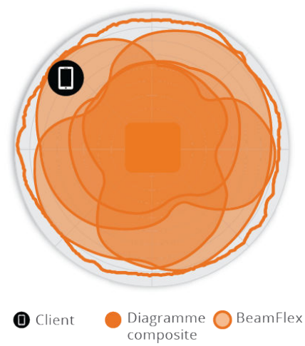
Figure 1. Exemple de diagramme BeamFlex
