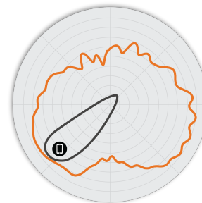
Figure 2. Diagrammes d'antennes Azimut R350 2,4 GHz Figure 3. Diagrammes d'antennes Azimut R350 5 GHz Figure 4. Diagrammes d'antennes Élévation R350 2,4 GHz Figure 5. Diagrammes d'antennes Élévation R350 5 GHz
