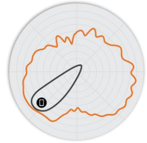
Figure 5. Diagrammes d'antennes Élévation R350 5 GHz
